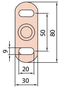
Frontansicht Typ B1 - B4
