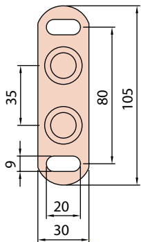
Frontansicht Typ F1 | F2
