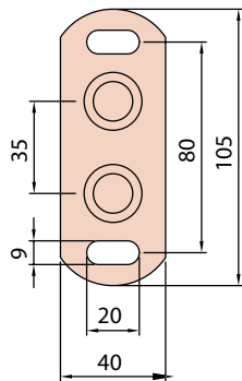
Frontansicht Typ F3 | F4
