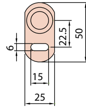
Frontansicht Typ C1 - C2
