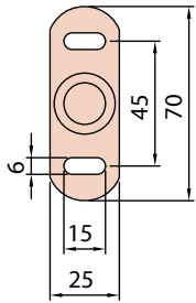
Frontansicht Typ A1 - A5
