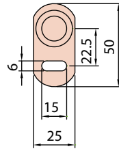
Frontansicht Typ C1 - C2
